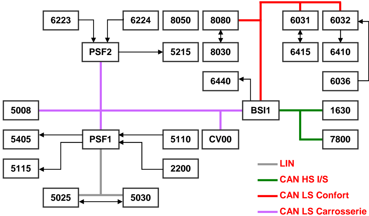
SCHEMA DES RESEAUX MULTIPLEXES
